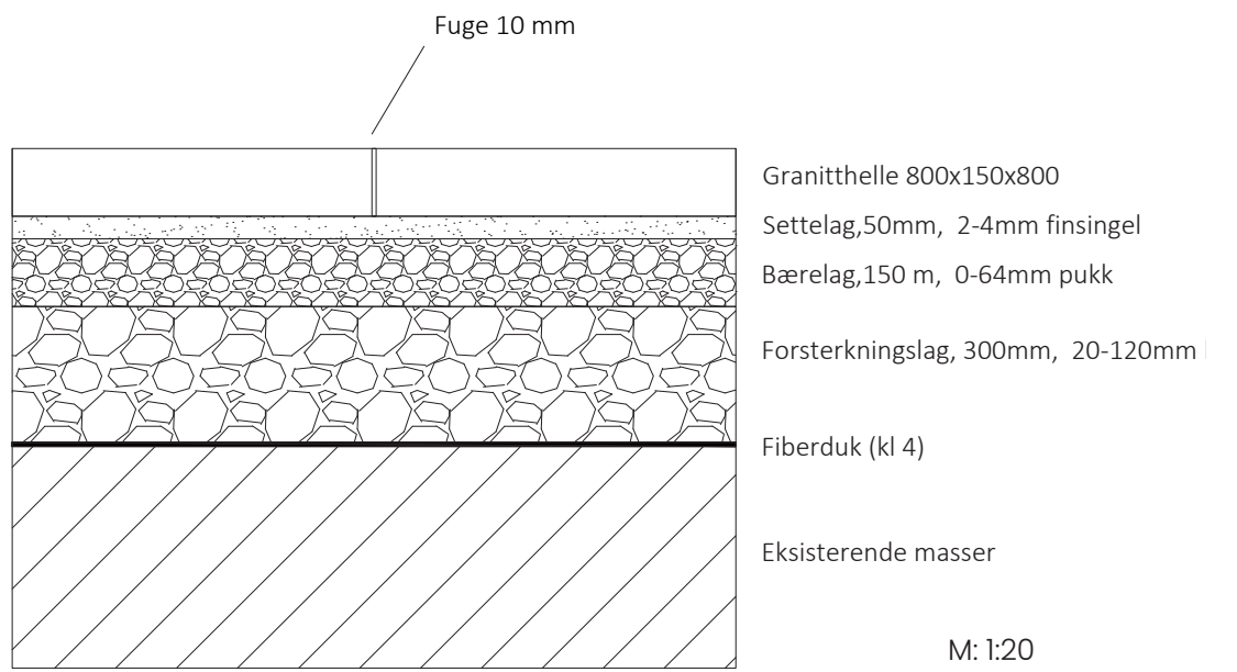
Prinsippskisse: fundamentering av granittbelegg utenfor fasadene
