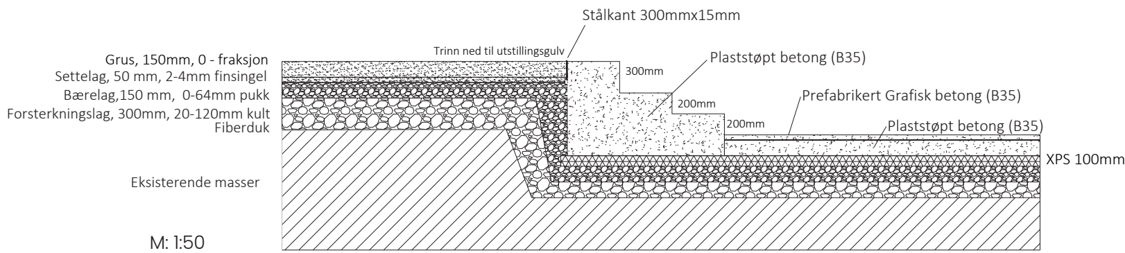
Prinsippskisse: fundamentering av grusdekke ved møte mot trinn i utstillingsgulvet.
