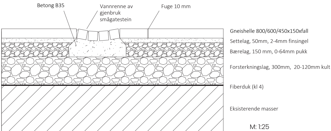
Prinsippskisse: fundamentering som viser til der vannrenne går gjennom belegg.
