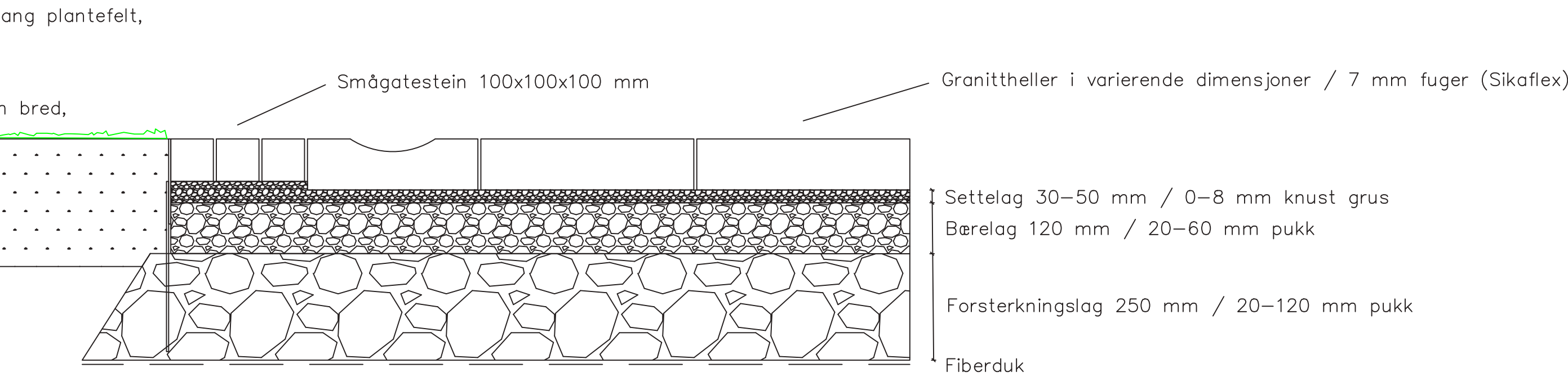
Prinsippsnitt av hvordan grøntareal møter cortenstål og steindekke. Vannrenna fanger opp overvann i nærheten av fasadene og fører vannet til et regnbed som samler, fordøyer og infiltrerer vannet videre.
