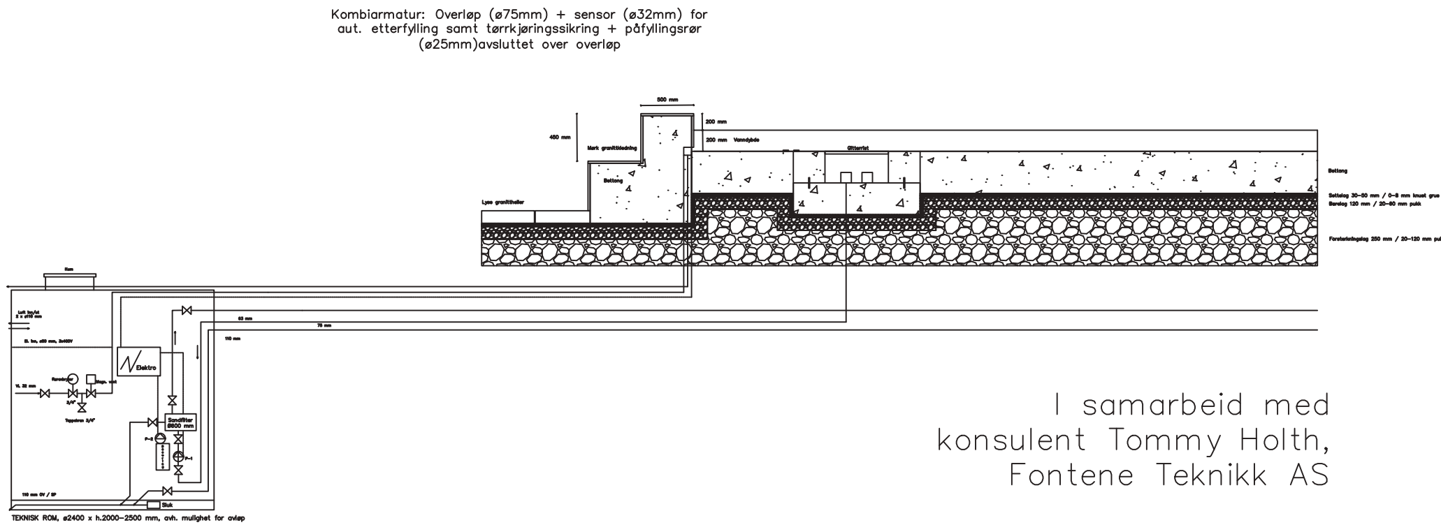
Prinsippsnitt av fundamenteringen til vannspeilet, med kobling til teknisk rom.
