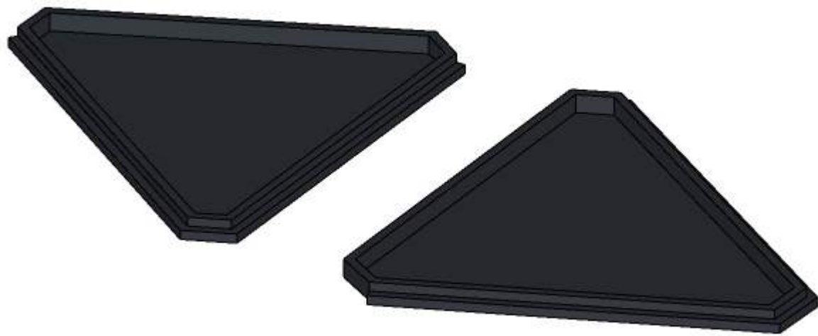
3D-modell av vannelementene i SketchUp. Sitteelementene går fra å være i flukt med terrenget, til å nå en sitte-høyde på 45 mm over terreng. Ok mur er på sitt høyeste 90 mm over terreng.
